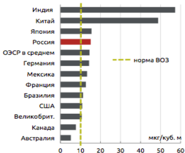
Рис. 1. Концентрация взвешенных частиц PM2.5 в среднем в 2015 г. по отдельным странам мира
